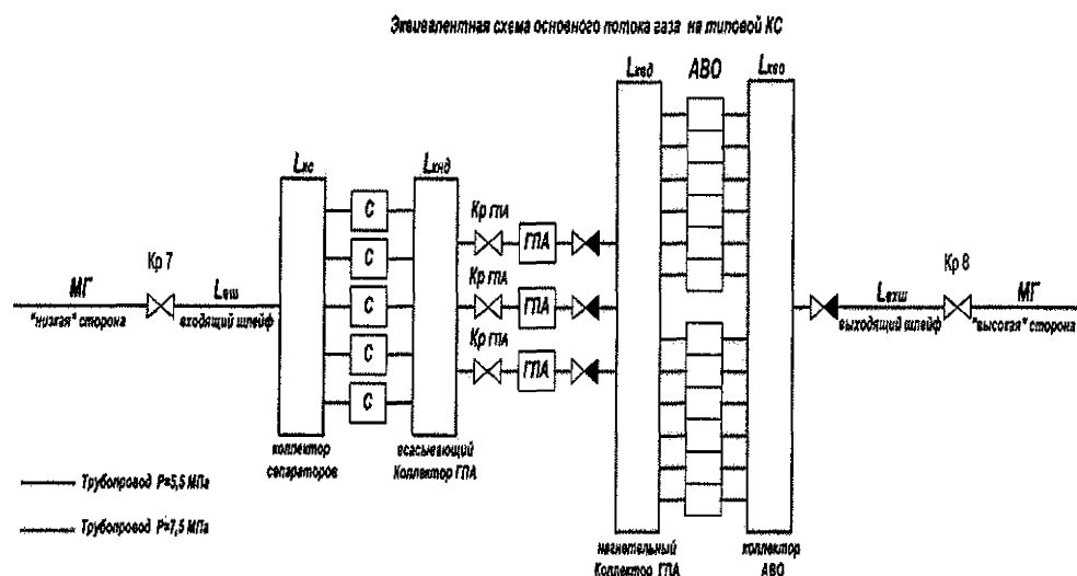
Рис. 4. Эквивалентная схема основного потока газа на типовой КС
