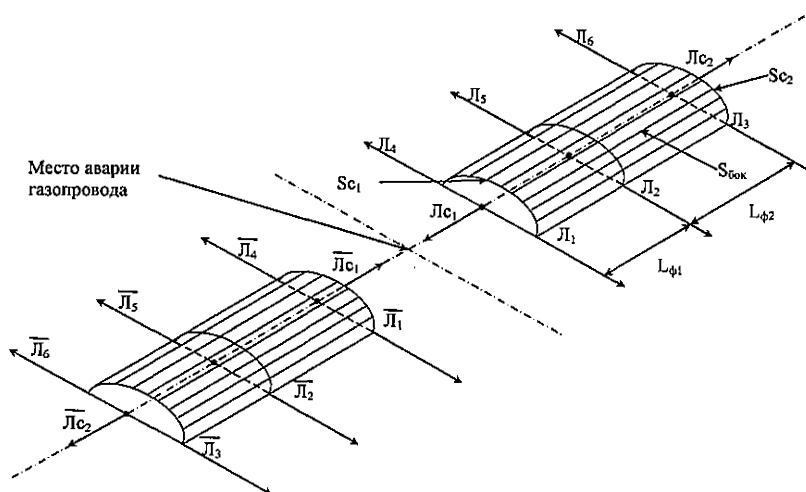
Рис. 7. Модель излучателя в виде двух полуцилиндров
