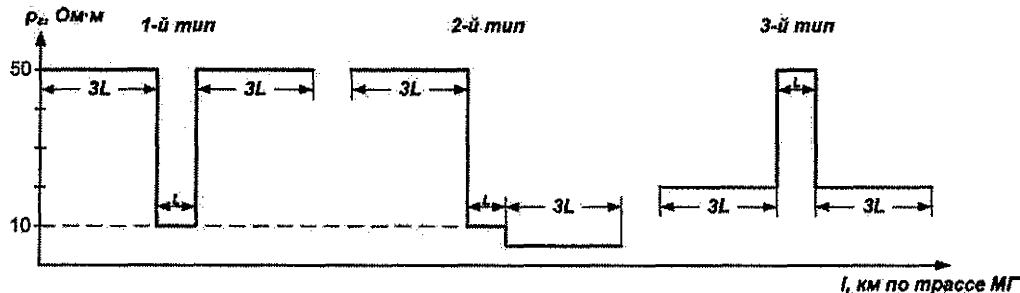
Рис. 1. Типы чередования грунтов с различными удельными сопротивлениями
