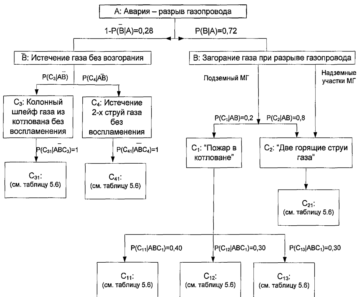
Рис. 1. Упрощенное дерево событий для идентификации сценариев аварий на МГ (здесь P(...|...) – условные вероятности реализации событий, указанных в блоках дерева (значения вероятностей приведены для МГ с Ду 1400мм))
