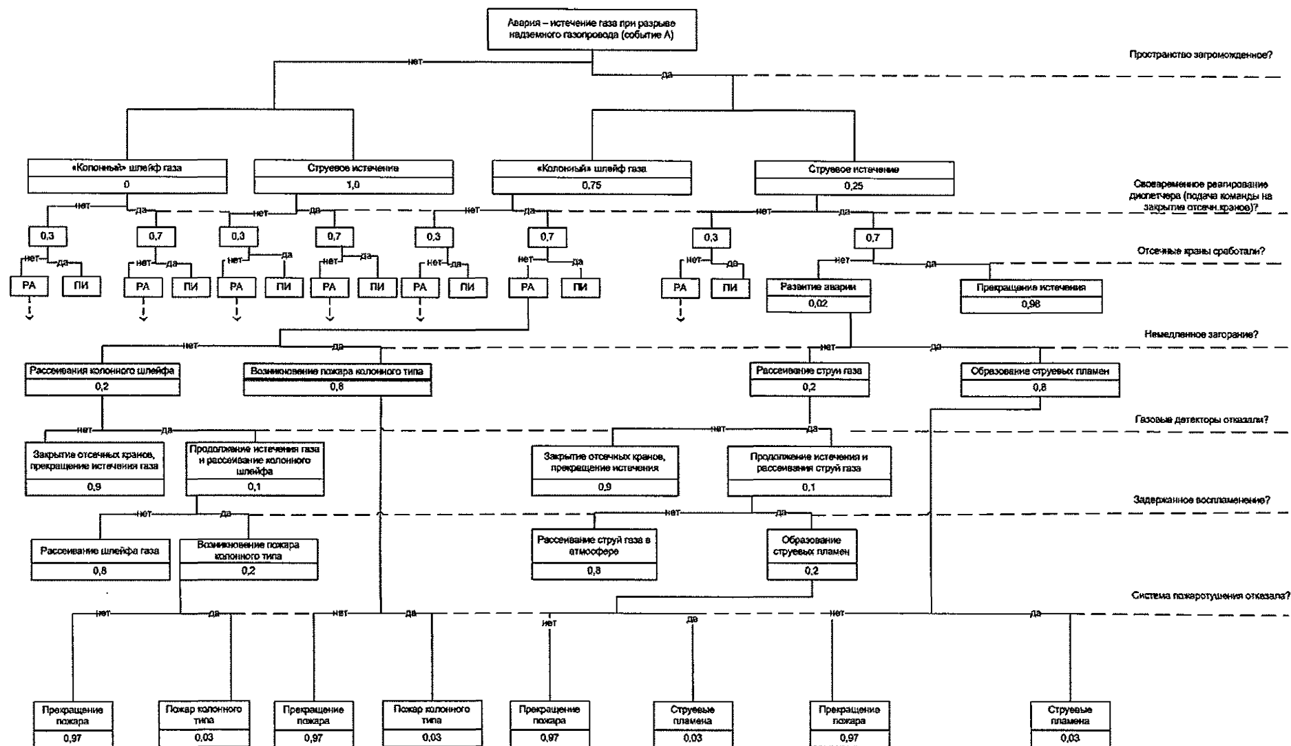
Рис. 4. Пример «дерева событий» (числа обозначают условные вероятности промежуточных событий, РА – развитие аварии, ПИ – прекращение истечения)
