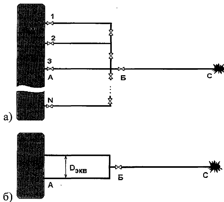
Рис. 3. Эквивалентная схема многопиточного газопровода для расчета аварийного истечения
